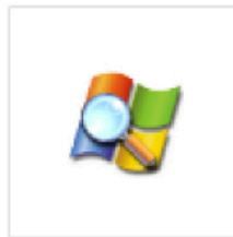
procexp.exe
