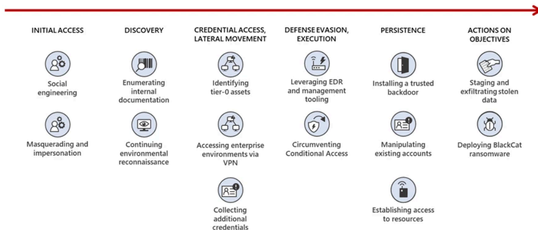
Figure 2. Octo Tempest TTPs
