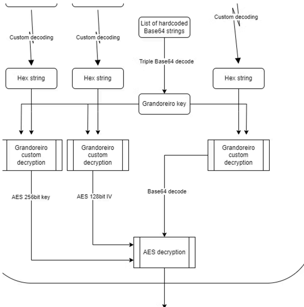
Fig 10: Grandoreiro loader string decryption
