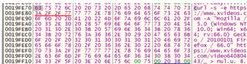
図20 curlコマンドの処理
