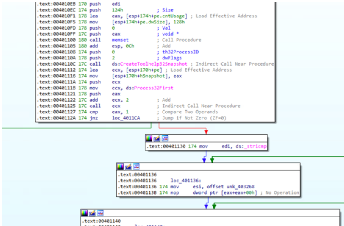
図15 プロセスチェックを行う処理
