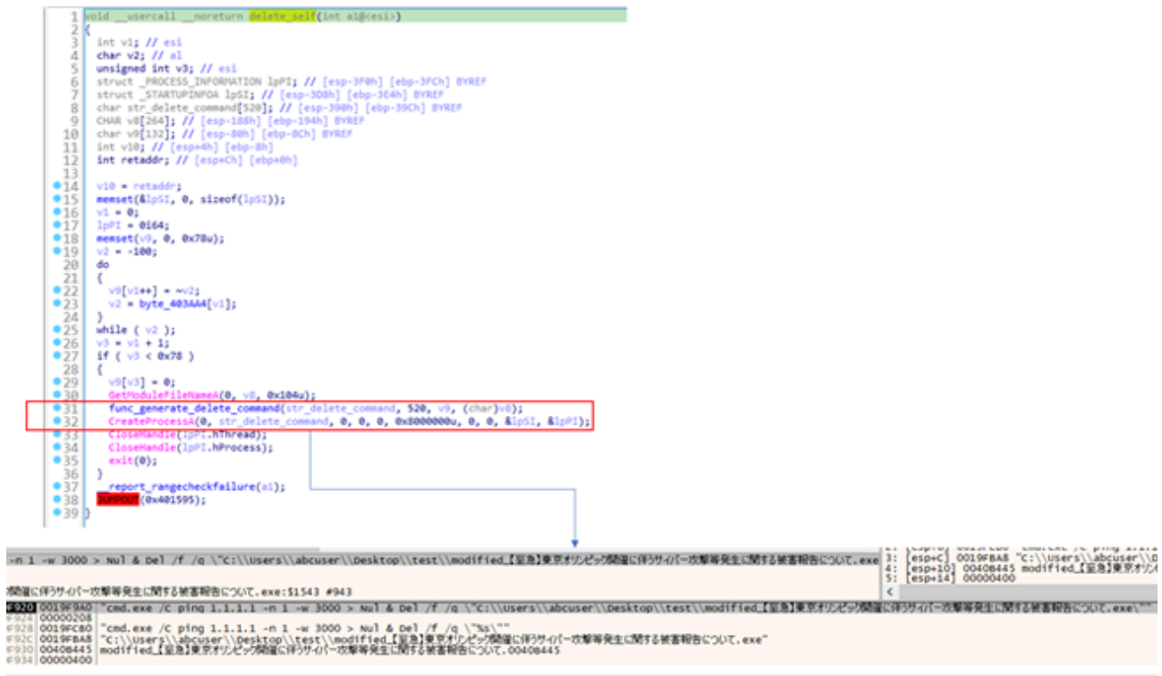
図21 自身を削除する処理
