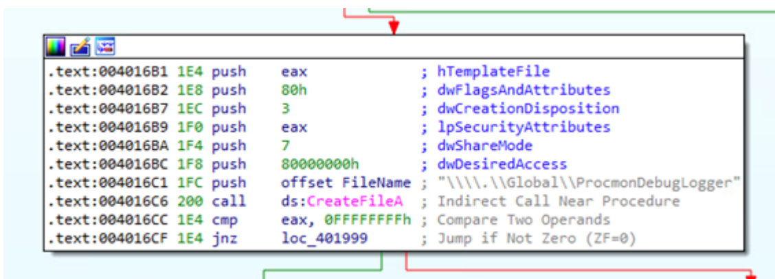
図16 Process Monitorに関するデバイスファイルの存在チェック
