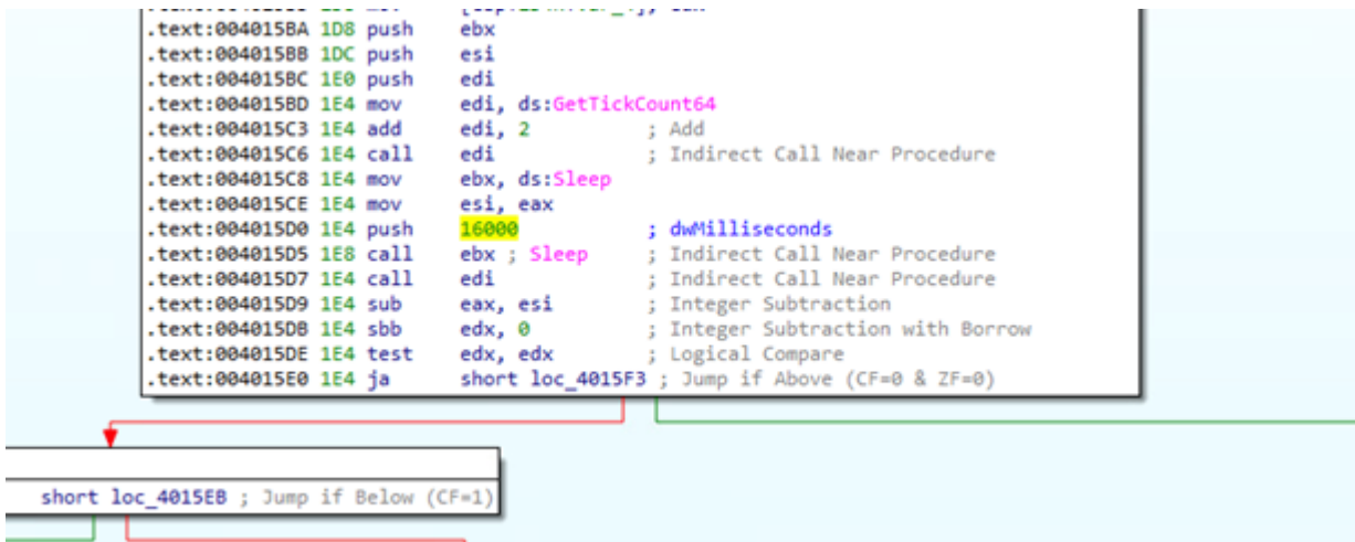
図7 GetTickCountによるコードの処理経過時間のチェック
